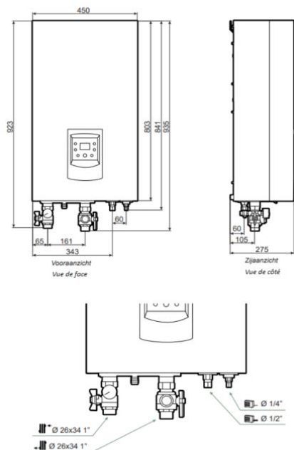
Besturingseenheid + opslageenheid
