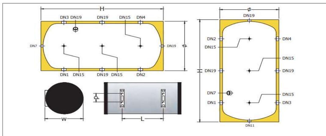
Afmetingen en aansluitingen
