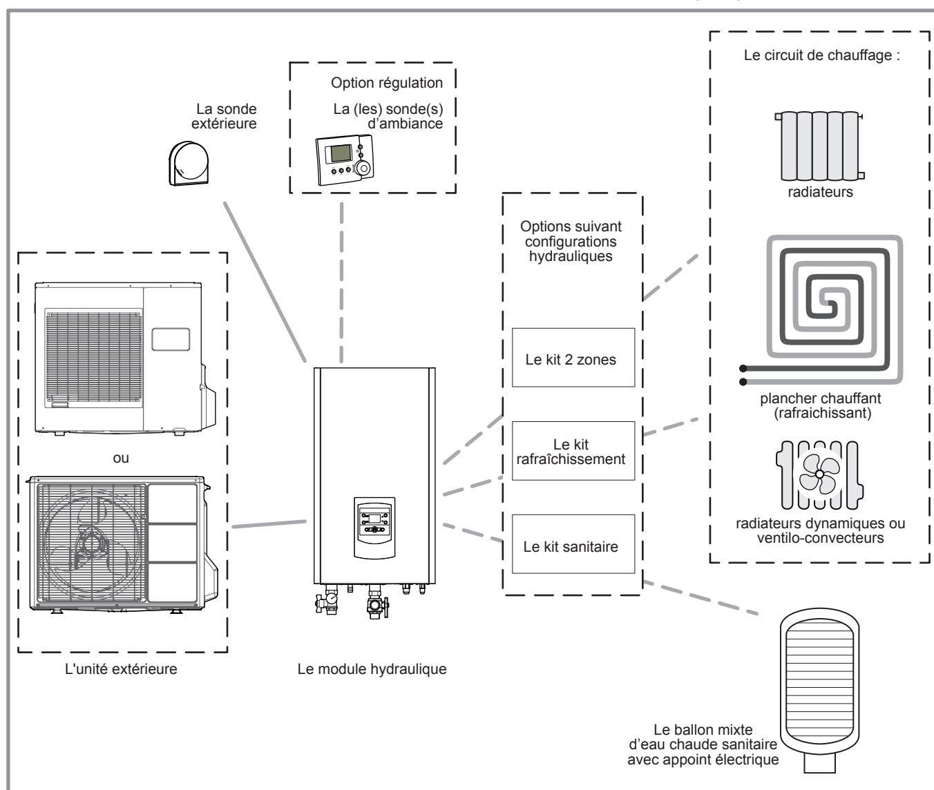
figure 1 - Vue d'ensemble d'une configuration d'installation complète
