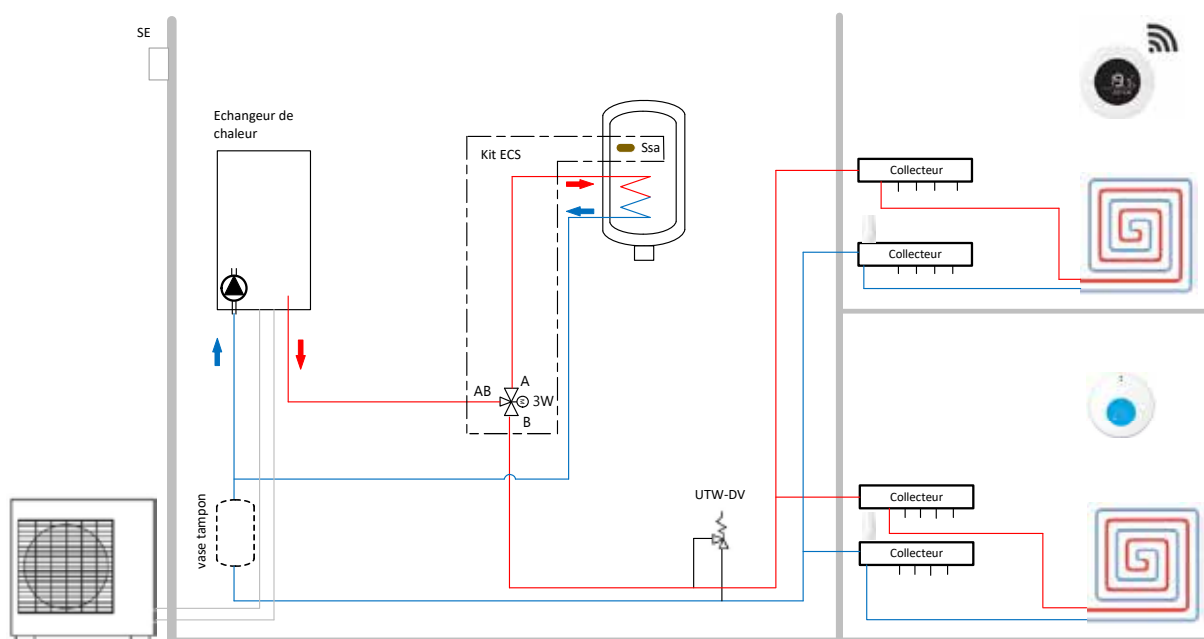
THERMA (Silent) Coax R410A Combi 1 circuit avec réglage par zone Adam
